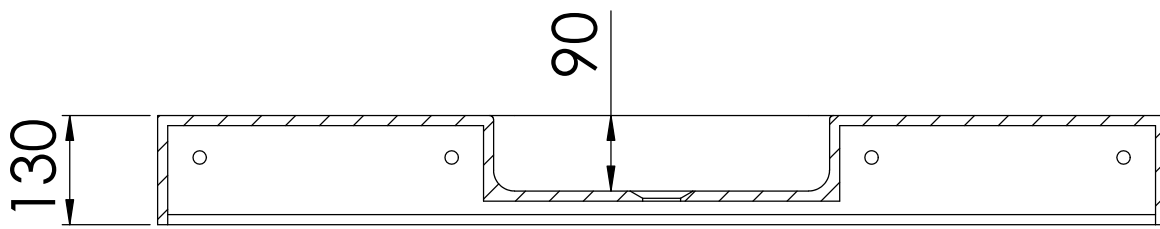
SCHNITT A-A
