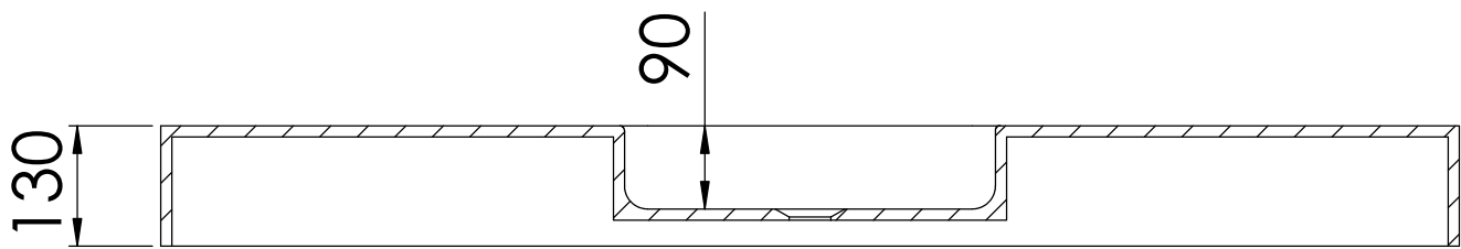
SCHNITT A-A
