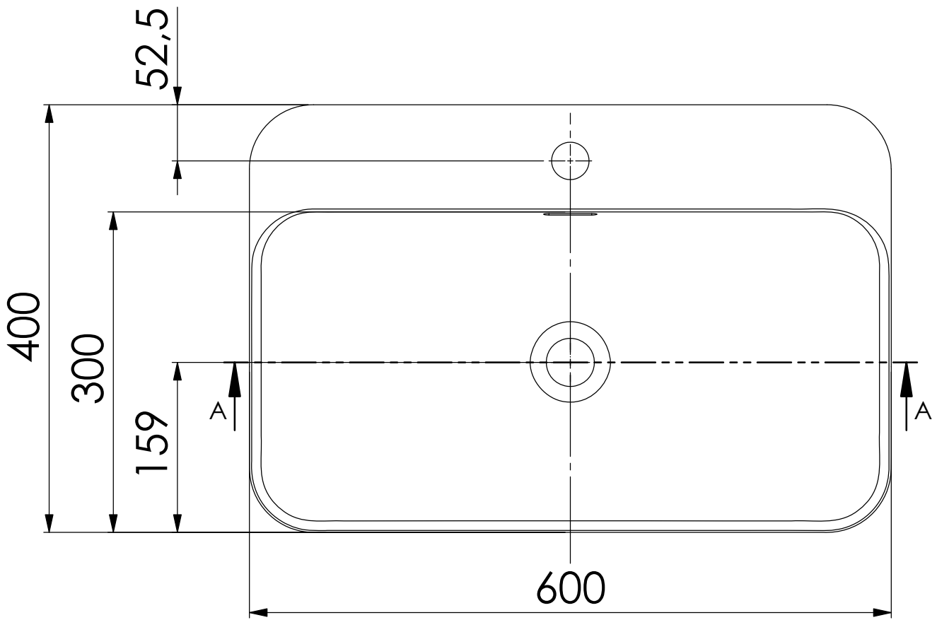
Schnitt A-A
