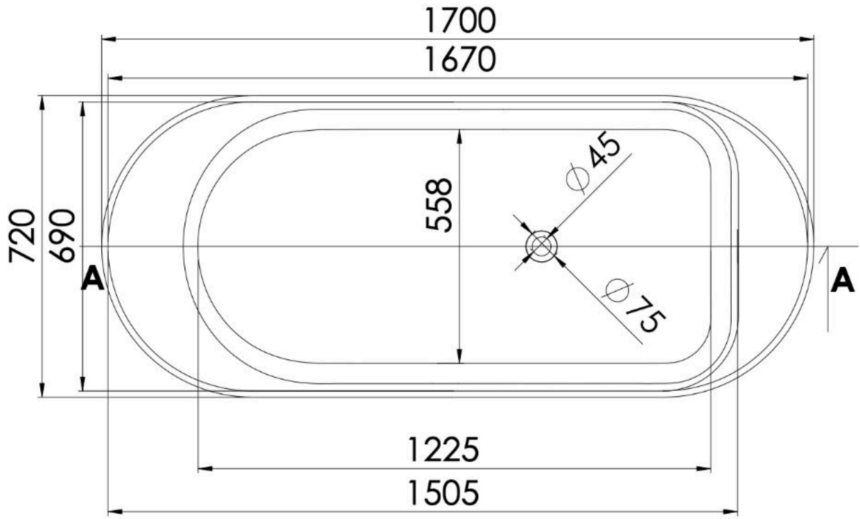
Schnitt A-A
